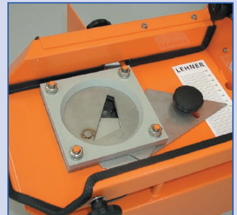
De doorgangshoeveelheid kan op de doseerschuif traploos worden ingesteld.
